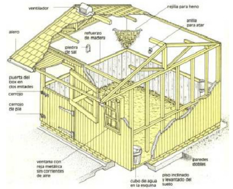
PERSPECTIVA CUADRA TIPO.
